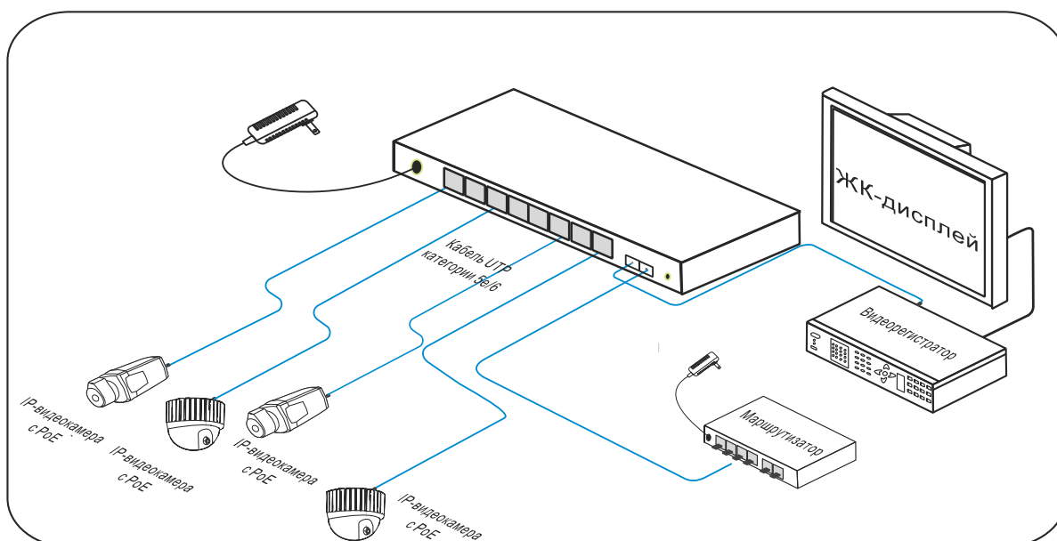
Рис. 3.2. Схема подключения оборудования к коммутатору
