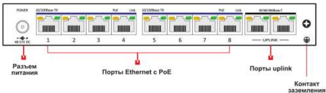
Рис. 2.2. Задняя панель
