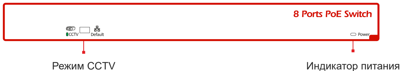
Рис. 2.1. Передняя панель
