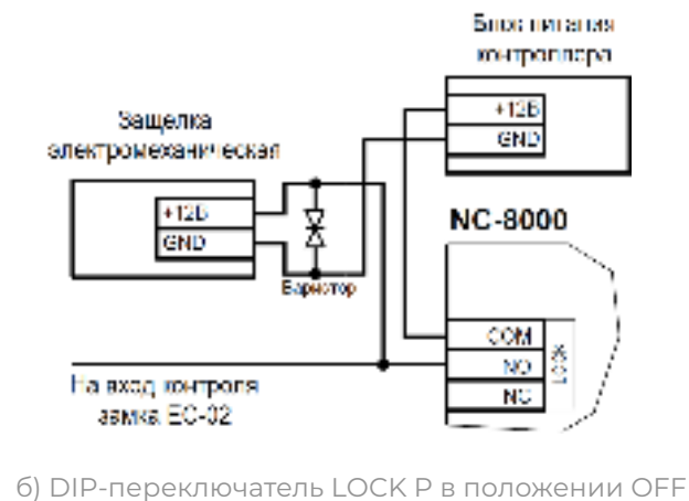
Рисунок 5. Контроль состояния замка, запираемого напряжением
