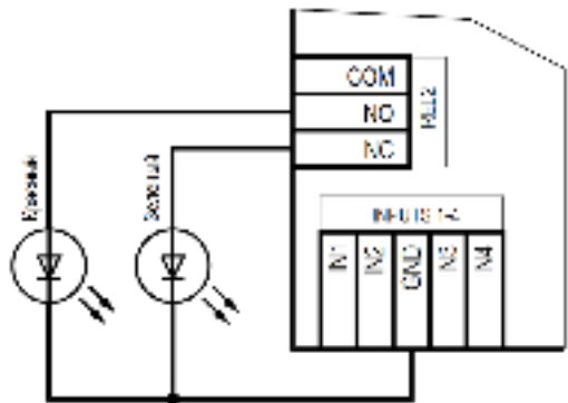
Рисунок 6. Подключение светодиодов
