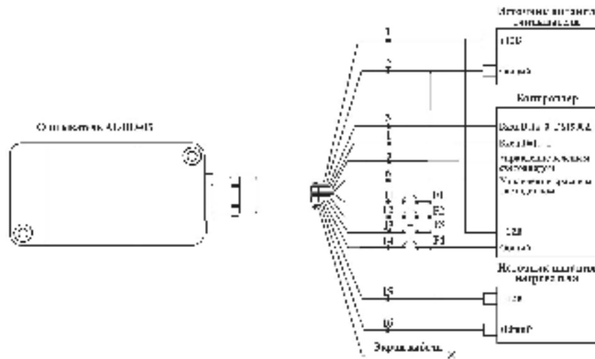
Рисунок 5 - Схема подключения считывателя AL-RD-05 к контроллеру СКВД с питанием считывателя от двух источников питания
