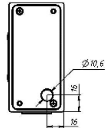
Рисунок 4 – Установочные размеры считывателя AL-RD-05 (вариант W)
