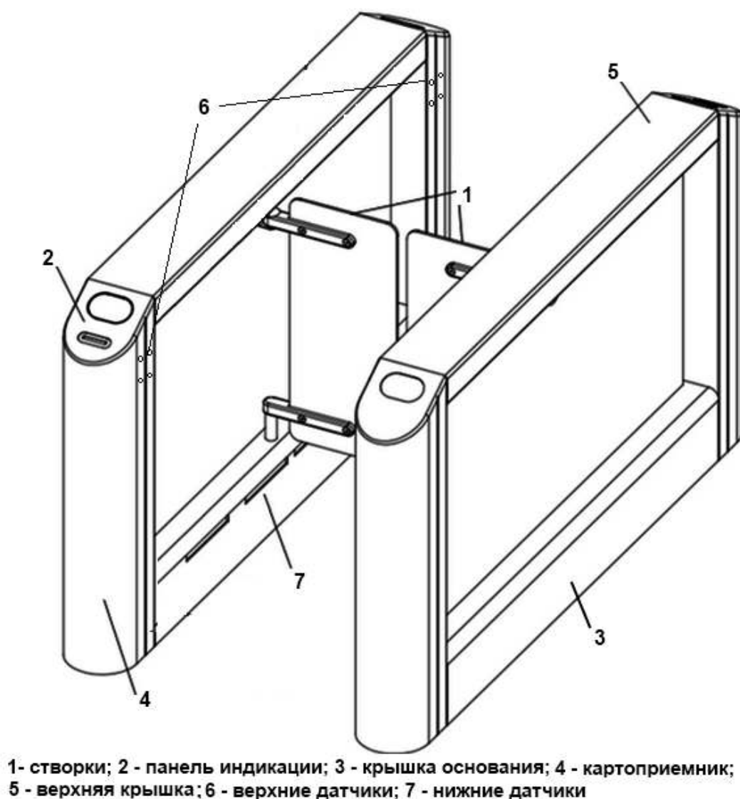
Рисунок 1 – Общий вид турникета
