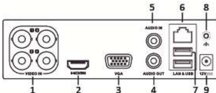
Рисунок 1.2 Задняя панель
