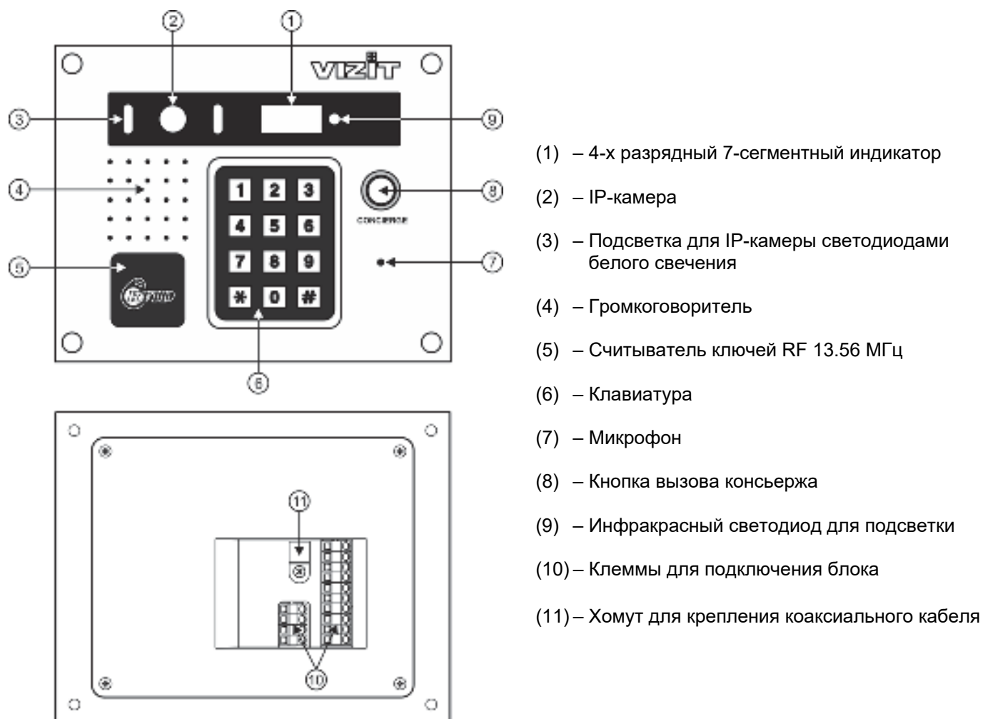
Рисунок 1.1 - Внешний вид блока вызова
