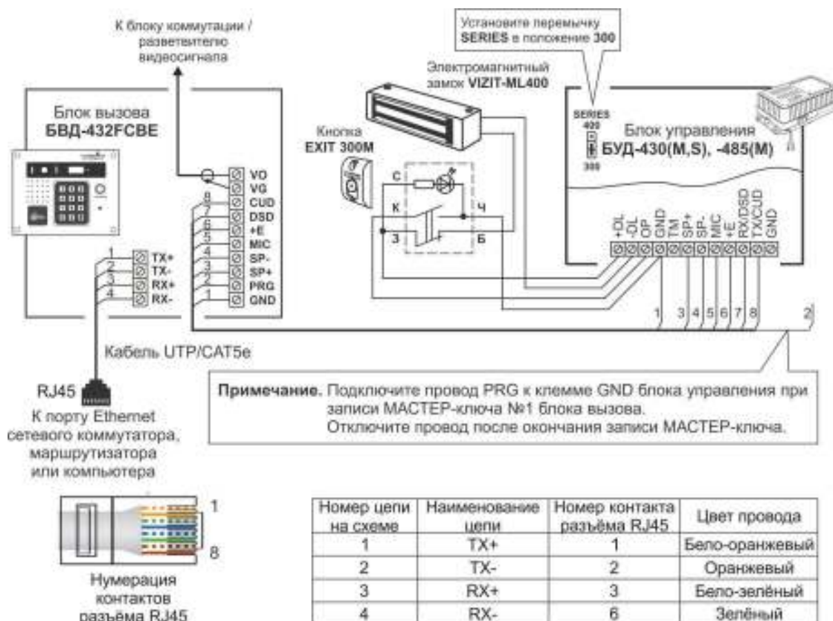
Рисунок 8.1 – Схема соединений блока вызова БВД-432ФСВЕ с блоком управления БУД-430(М,С), -485(М), электромагнитным замком VIZIT-ML400 и кнопкой EXIT 300М
