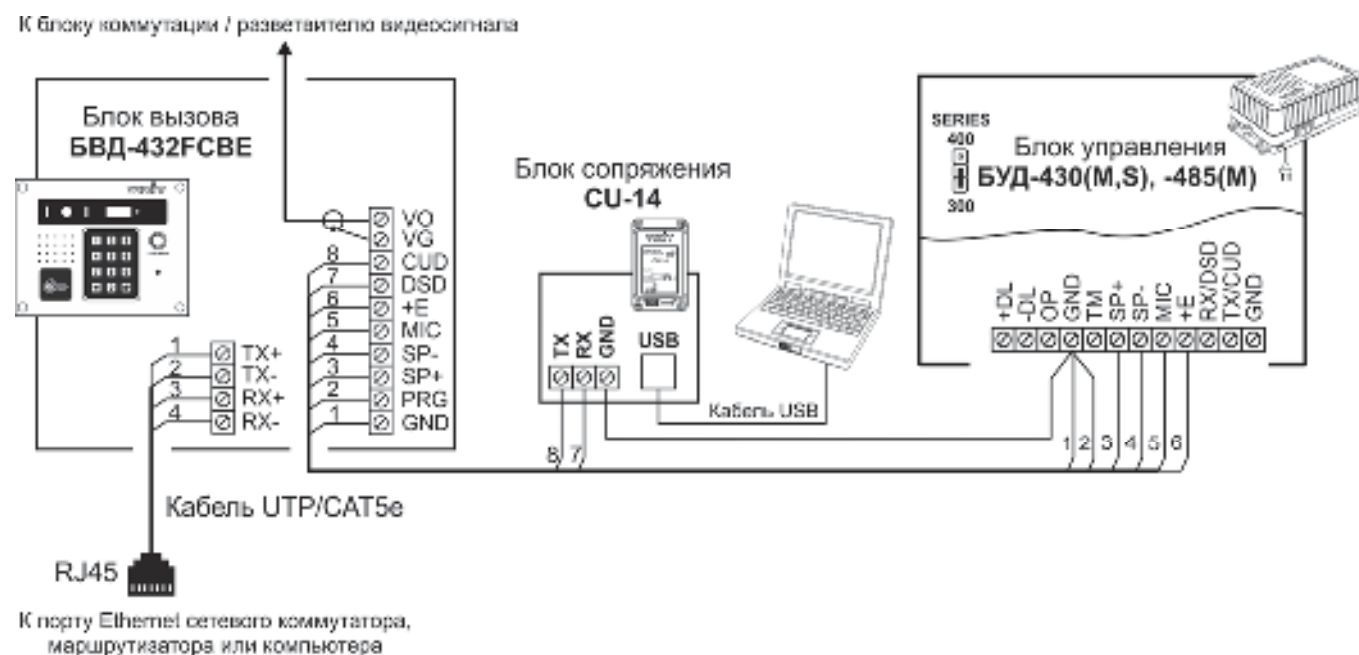
Рисунок 15.1 - Схема соединений блока вызова с блоками управления БУД-430(S, М), -485(М) и блоком сопряжения CU-14
