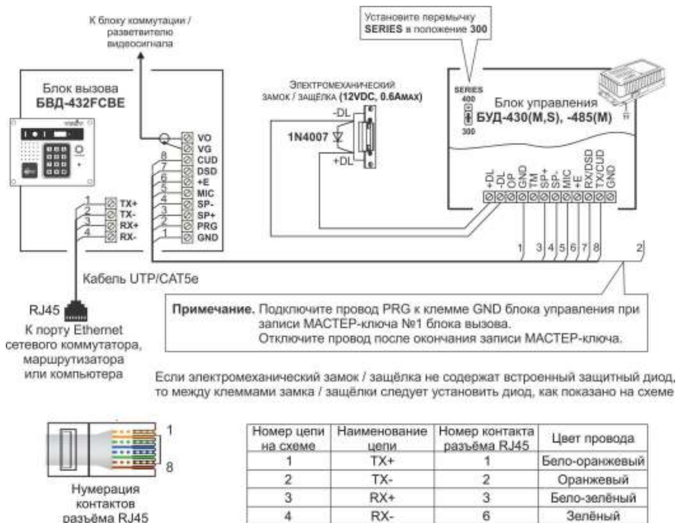
Рисунок 8.3 – Схема соединений блока вызова БВД-432FCBE с блоком управления БУД-430(М,С), -485(М) и электромеханическим замком / защёлкой
