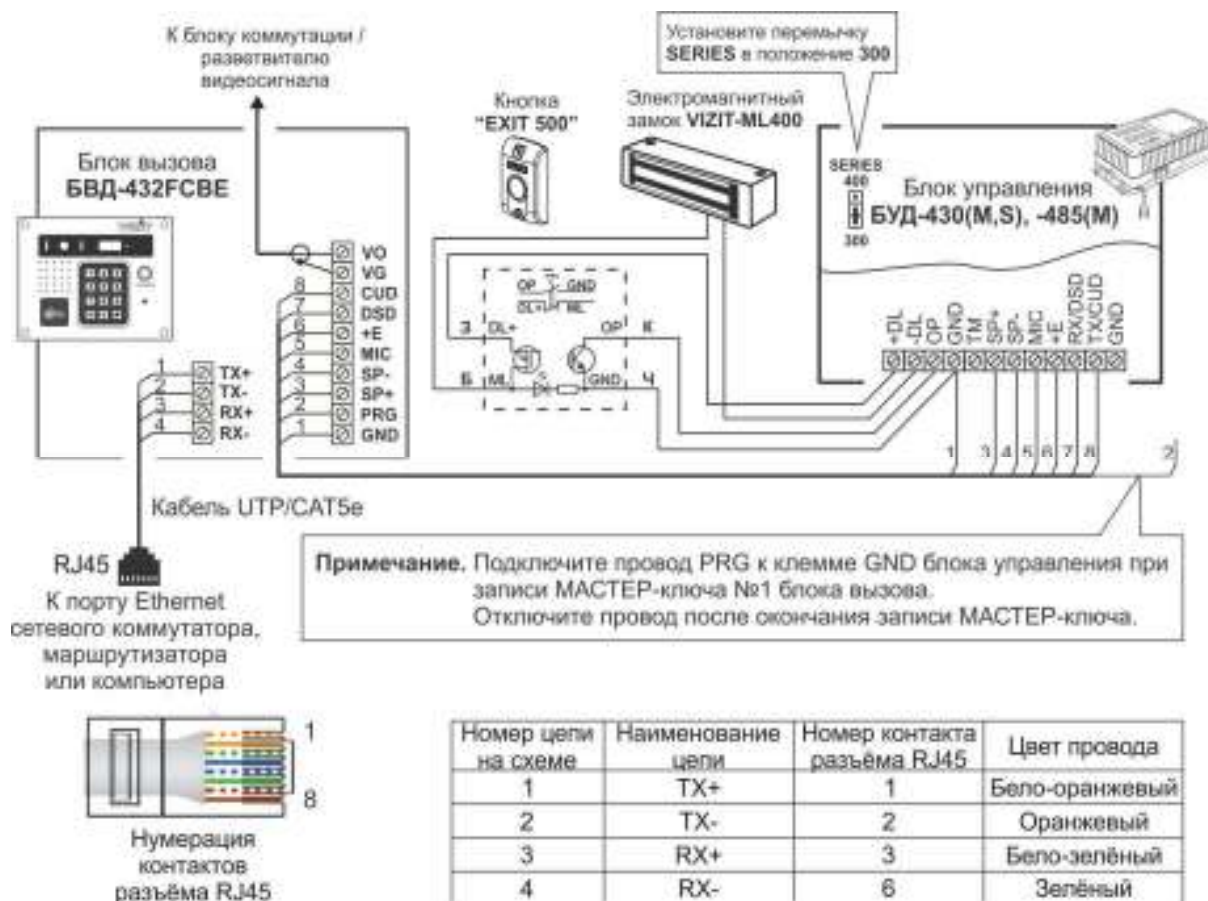
Рисунок 8.2 – Схема соединений блока вызова БВД-432ФСВЕ с блоком управления БУД-430(М,С), -485(М), электромагнитным замком VIZIT-ML400 и кнопкой EXIT 500
