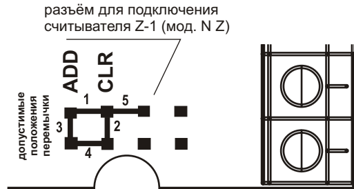
Рис. 3 Положения перемычки
