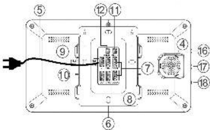
Конструкция монитора
