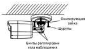
Рисунок 2-2 Установка камеры на потолок
