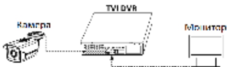
Рисунок 3-1 Подключение
