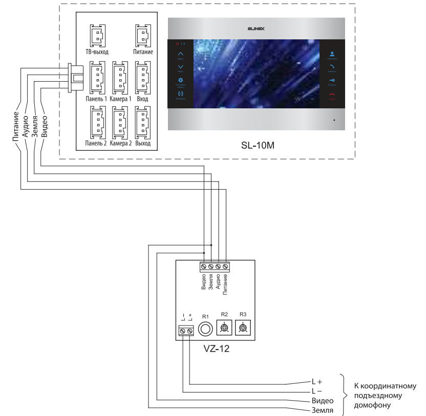
Схема подключения адаптера VZ-12
