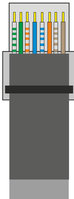
Рис. 5.1. Разводка проводов по стандарту EIA/TIA 568A
