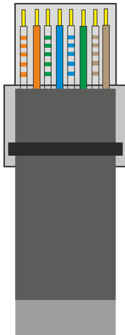
Рис. 5.2. Разводка проводов по стандарту EIA/TIA 568B
