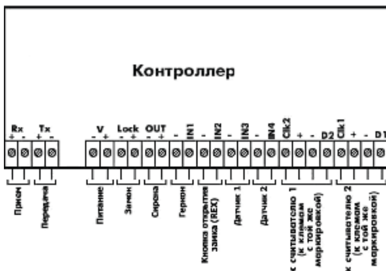
Рисунок 3 – Одна дверь, два считывателя
