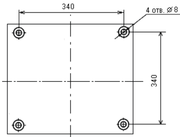
Рисунок 10 – Крепление контроллера (присоединительные размеры)
