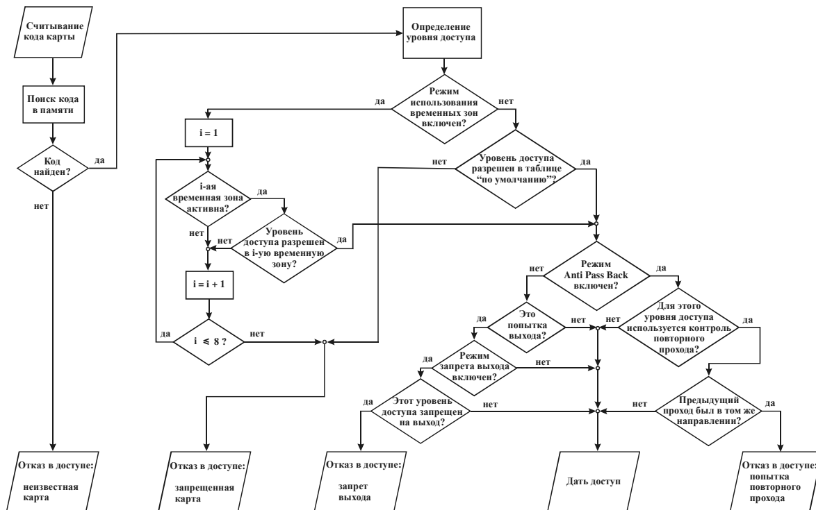
Рисунок 11 – Схема принятия решения о допуске
