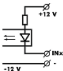
Рисунок 5 – Схема входных каскадов “Inx”
