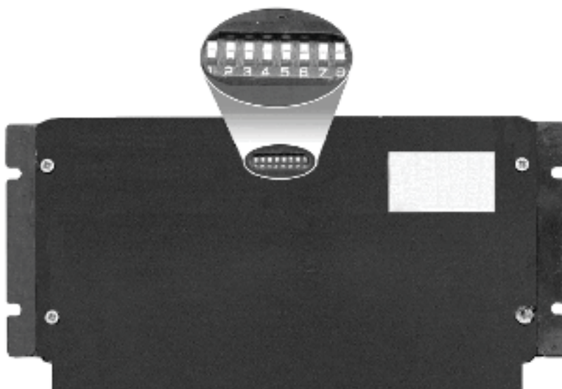
Рисунок 7 – DIP-переключатели контроллера
