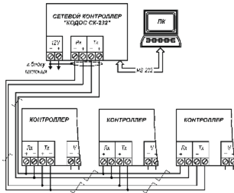
Рисунок 9 – Схема подключения контроллеров к сетевому контроллеру «КОДОС СК-232». Связь с сетевым контроллером «КОДОС СК-Е» осуществляют по аналогичной схеме
