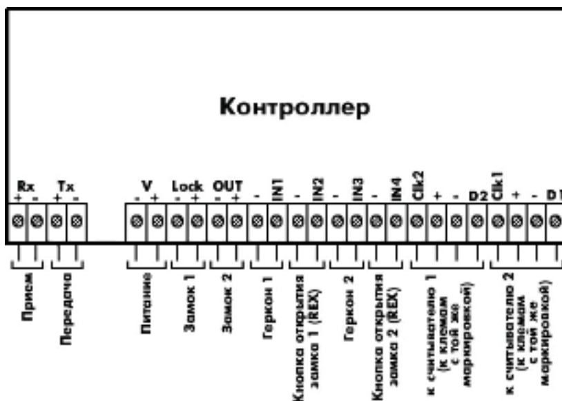
Рисунок 4 – Две двери, два считывателя
