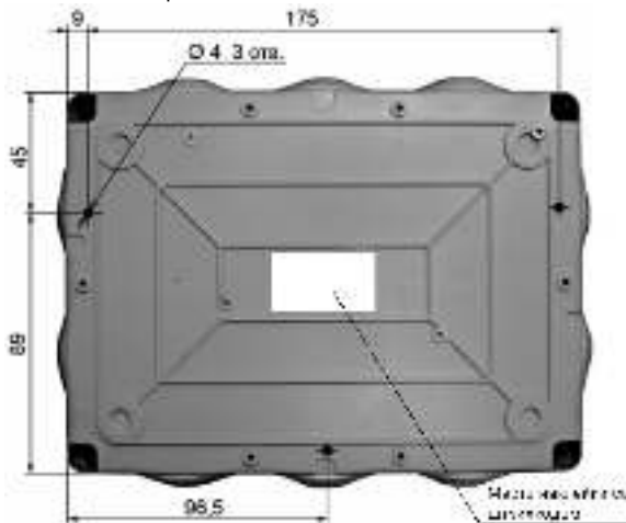
Рисунок 4 - Крепление контроллера (установочные размеры)
