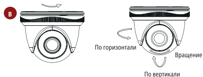
Рис. 4 Установка камеры НТ 12 | НТ 22 | НТ 52 на потолок
