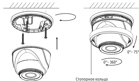
Рис. 6 Установка камеры НТ 27
