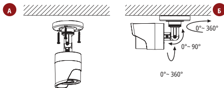
Рис. 5 Установка камеры НТ 13|НТ 23|НТ 53 на потолок
