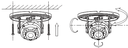
Рис. 1 Установка камеры HIT 10|HIT 20 на потолок
