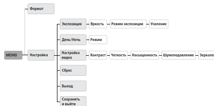
Рис 10 Общий вид меню.
