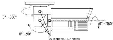
Рис. 6 Регулировка угла обзора камеры НИТ 28|НИТ 58
