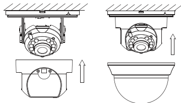
Рис. 2 Установка камеры HIT 10 | HIT 20 на потолок
