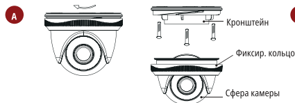
Рис. 3 Установка камеры HIT 12 | HIT 22 | HIT 52
