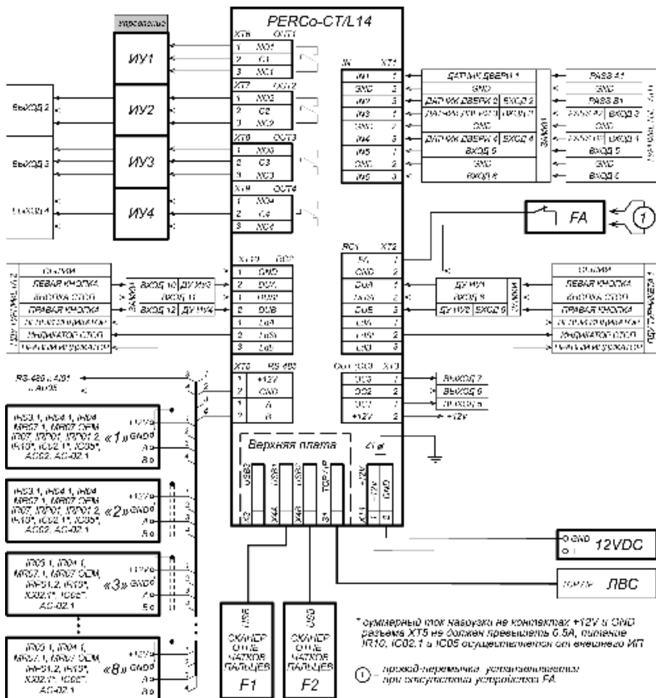
Рисунок 3. Общая схема подключений
