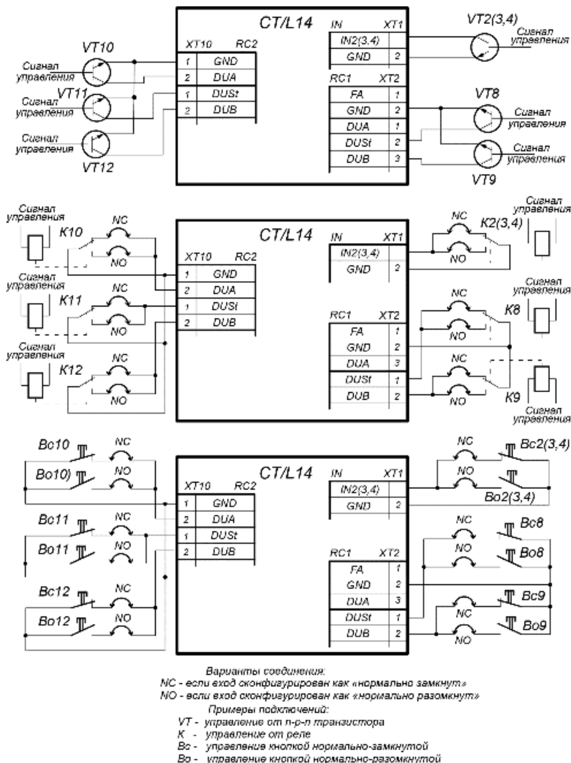
Рисунок 13. Схема подключений доп. оборудования к входам контроллера
