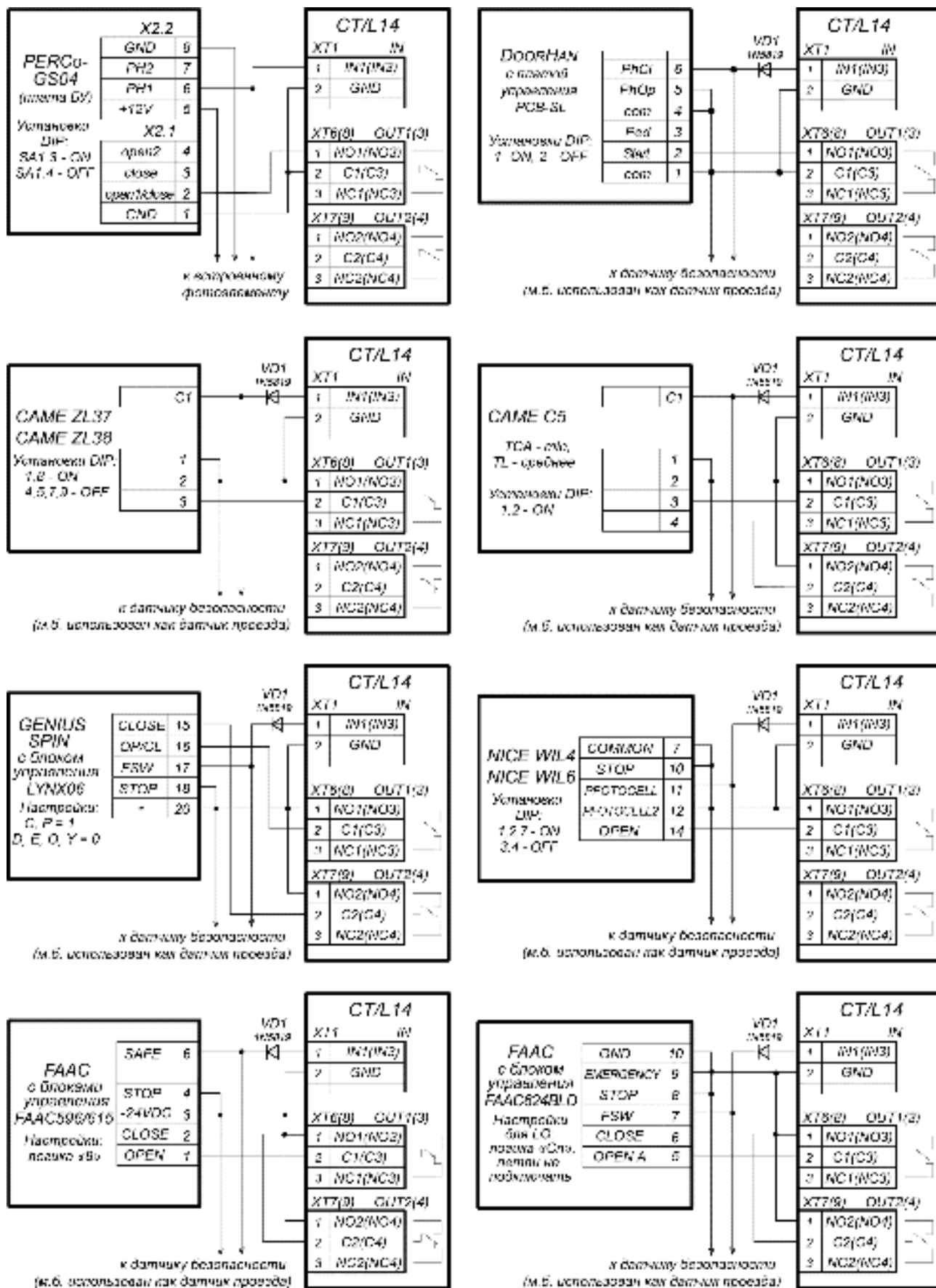
Рисунок 8. Примеры схем подключения шлагбаумов к контроллеру АТП
