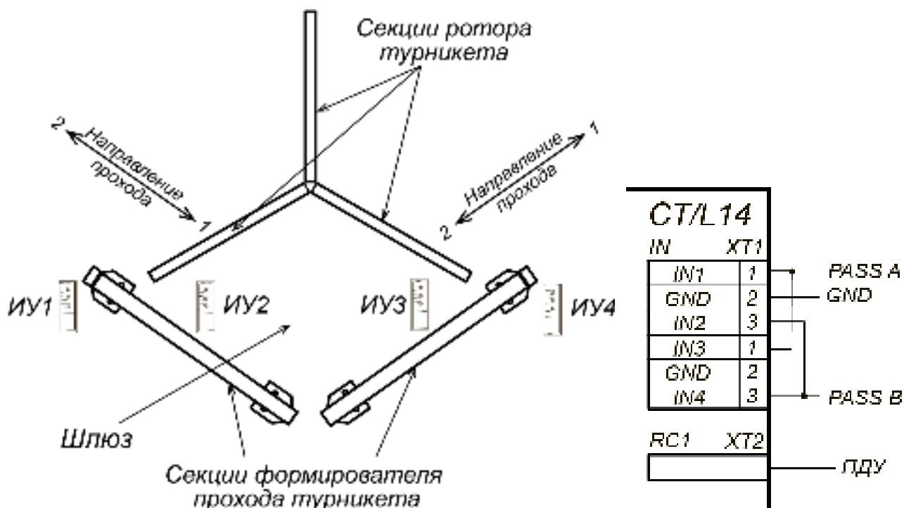
Рисунок 23. Схема шлюза из роторного турникета
