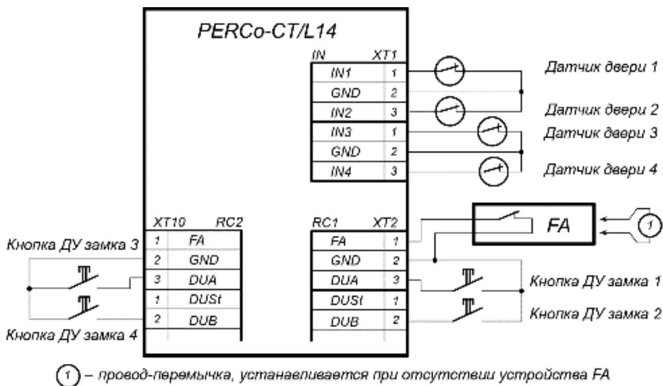
Рисунок 5. Схема подключений кнопок ДУ и датчиков двери
