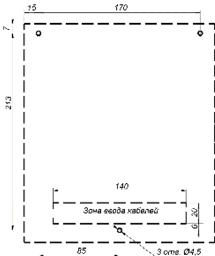
Рисунок 2. Разметка отверстий для монтажа контроллера
