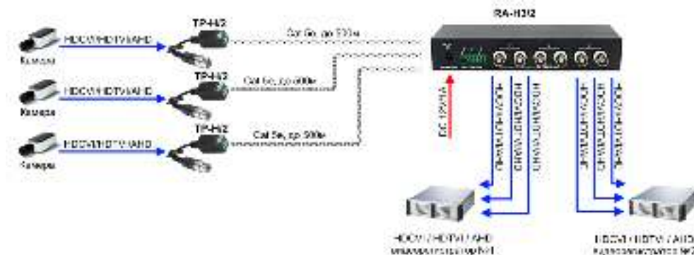
Рис.3 Схема подключения активного приемника RA-H3/2 в комплекте с пассивными приемопередатчиками TP-H/2
