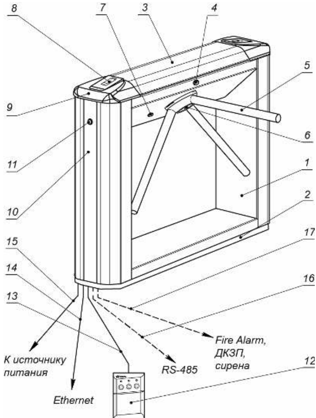
Рисунок 1. Устройство ЭП
