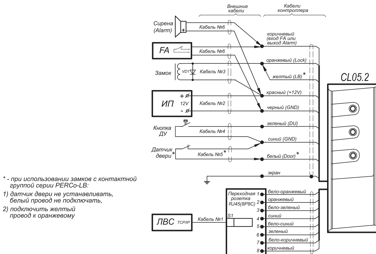
Схема подключений контроллера CL05
