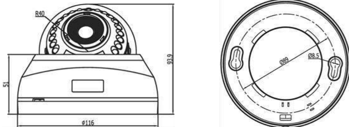
Рис. 1.2. Размеры видеокамеры, мм
