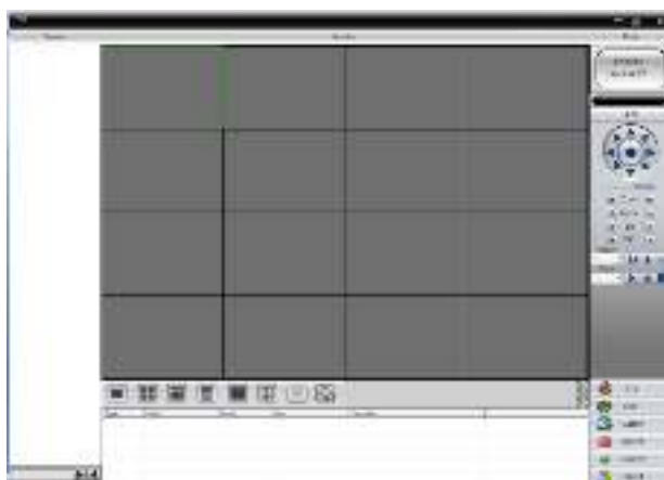
Рис. 2.6 CMS интерфейс
