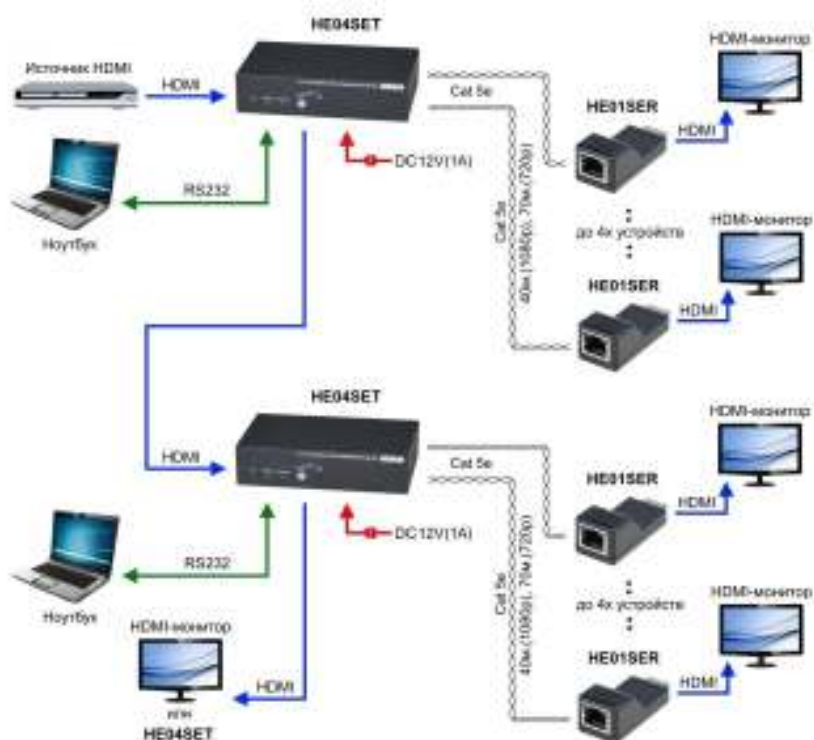
Рис.7 Схема каскадного подключения комплектов HE04SEK
