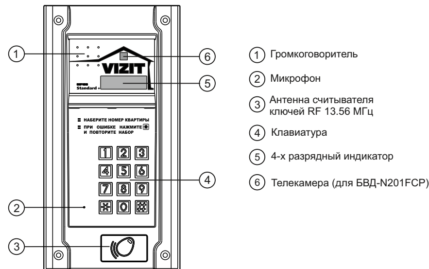
Рисунок 1 - Внешний вид блока вызова
