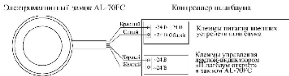
Рисунок 5 - Схема подключения замка
