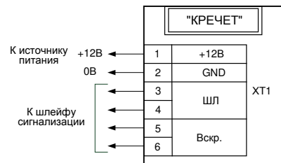
Рисунок 2 Схема подключения извещателя «Кречет»
