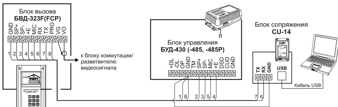
Рисунок 14 - Схема соединений блока сопряжения с блоками управления БУД-430 (-485, -485Р)
