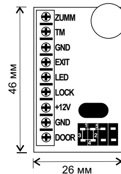
Рис.1 Внешний вид и габаритные размеры платы
