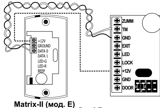
Рис. 3 Подключение внешнего считывателя
