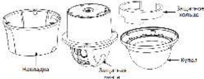
Рисунок 1-16 Демонтаж камеры
