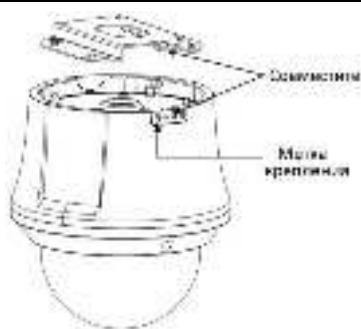
Рисунок 1-18 Установка камеры на потолок
