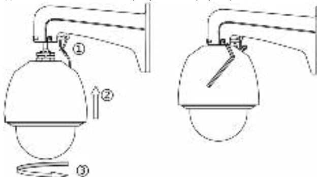
Рисунок 1-8 Установка скоростной поворотной камеры
