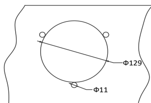
Рисунок 1-9 Шаблон крепления
