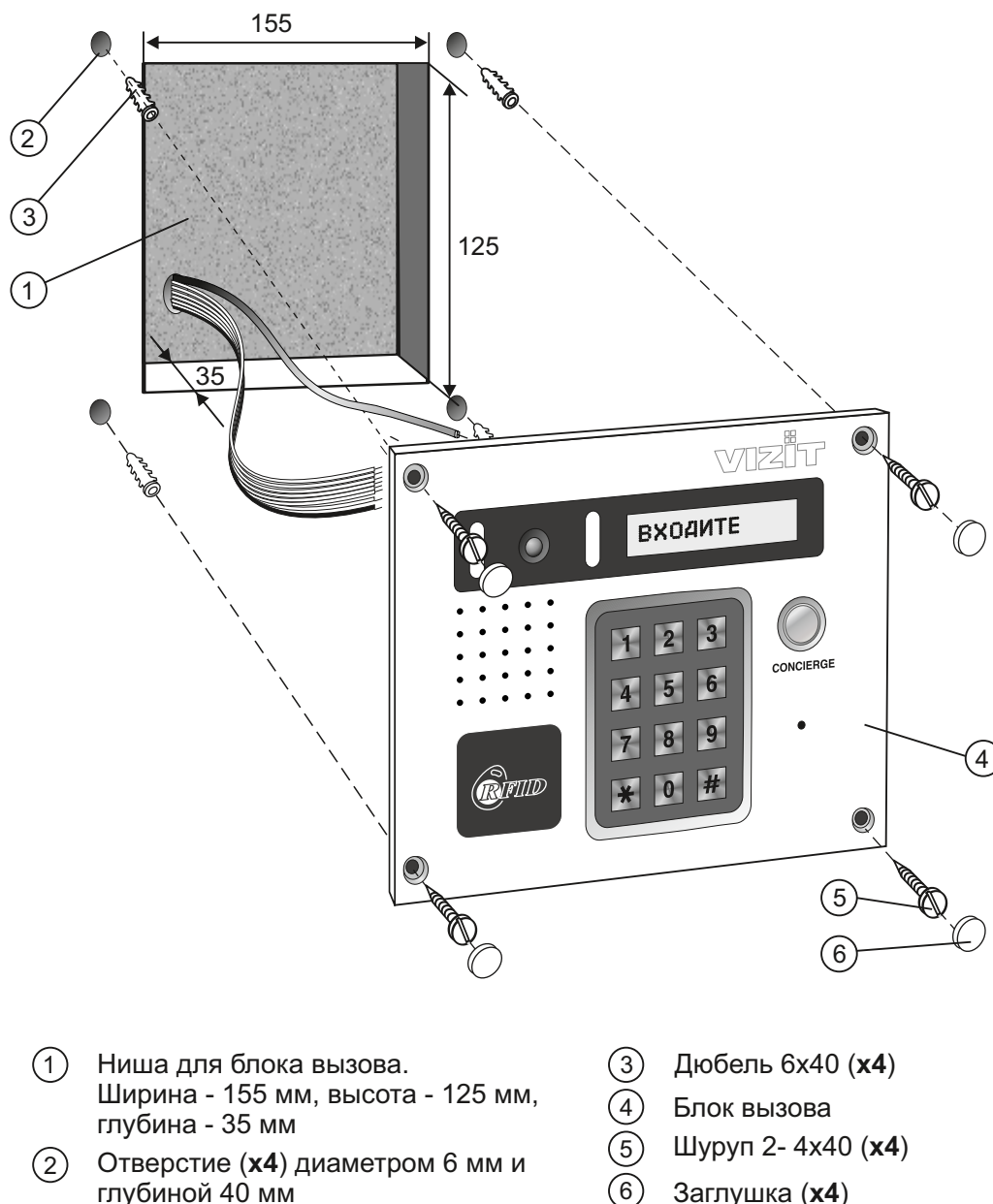
Рисунок 2 - Установка блока на стену
