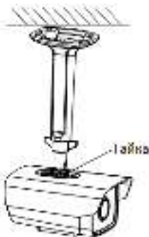
Рисунок 2-6 Установка камеры на монтажный кронштейн
