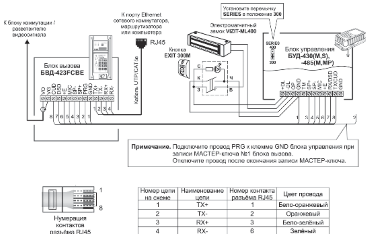
Рисунок 8.1 – Схема соединений блока вызова БВД-423FCBE с блоком управления БУД-430(M,S), -485(M,MP), электромагнитным замком VIZIT-ML400 и кнопкой EXIT 300M
