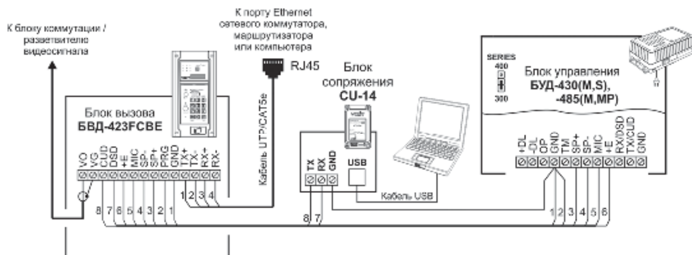
Рисунок 15.1 - Схема соединений блока вызова с блоками управления БУД-430(S, М), -485(М, МР) и блоком сопряжения CU-14
