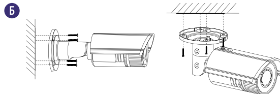
Рис. 20 Установка камеры PRO x8
