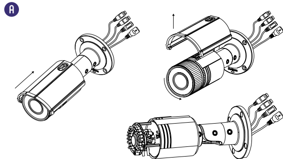
Рис. 19 Настройка зума и фокуса PRO x8
