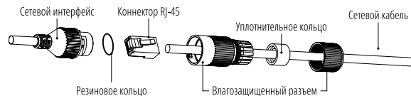
Рис. 10. Сетевой влагозащищенный разъем
