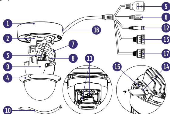
Рис. 5 Описание камеры PRO ×7
