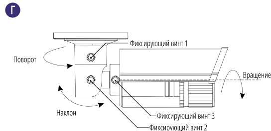
Рис. 21 Установка камеры PRO x8
