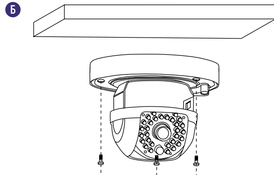
Рис. 12 Установка камеры PRO x4
