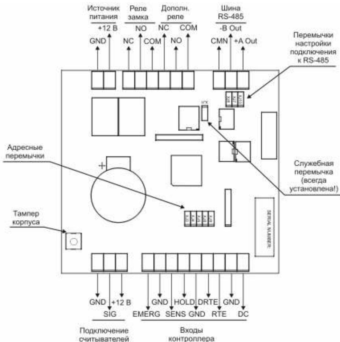
Рисунок 3. Печатная плата контроллеров NC-2000-D.
