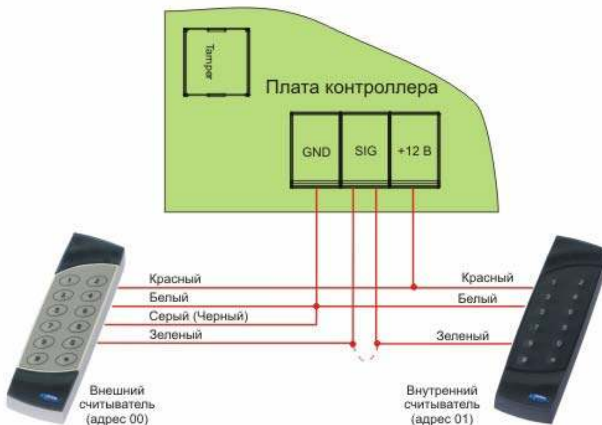
Рисунок 5. Подключение считывателей серии NR-xxx к контроллерам NC-2000-D.
