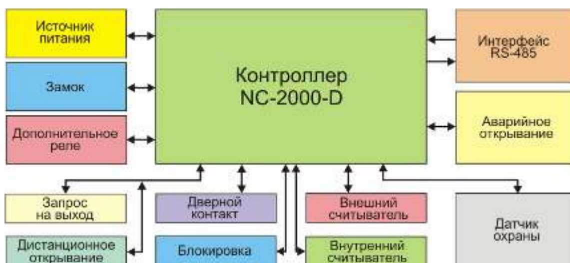
Рисунок 4. Оборудование, подключаемое к контроллерам NC-2000-D.
