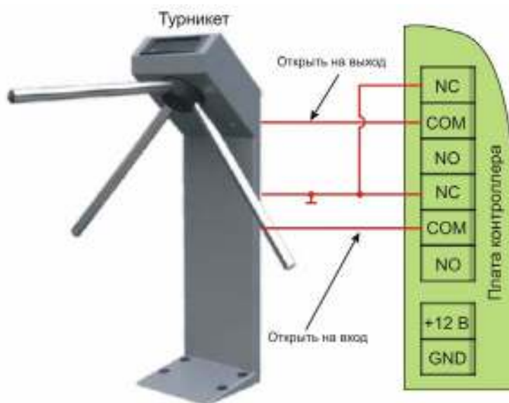
Рисунок 10. Подключение контроллера к турникету.
