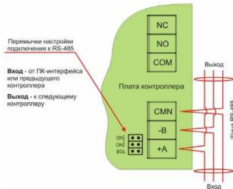
Рисунок 16. Подключение контроллера к шине RS-485.
