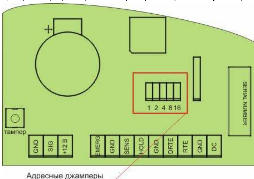
Рисунок 17. Установка адресных джамперов.
