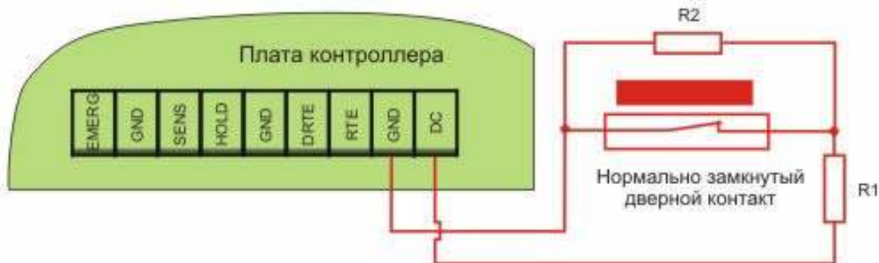
Рисунок 76. Подключение DC с контролем подводящих проводов.
