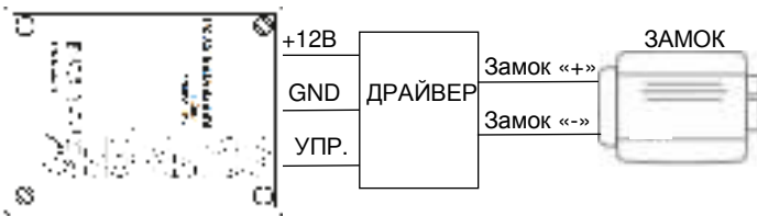
Рисунок 1 — Схема подключения драйвера
