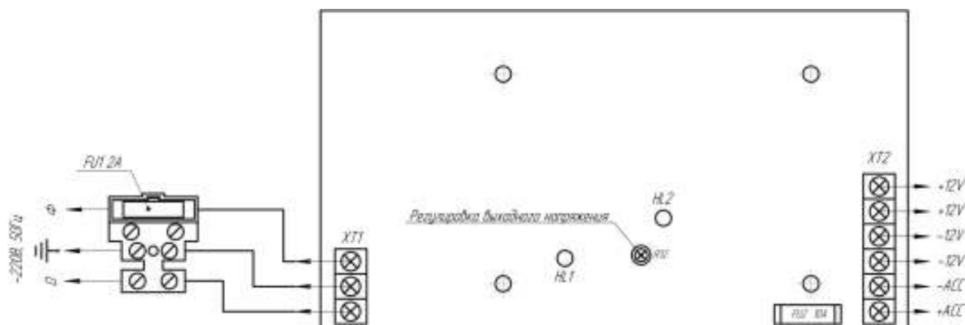
Рис. 1 Схема подключения
