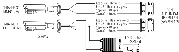
Рис. 9 Схемы подключения видеокamеры к монитору MAGIC HD
