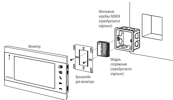
Рис. 4 Монтаж монитора видеодомофона MAGIC
