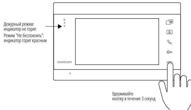
Рис. 11 Быстрая активация|деактивация режима "Не беспокоить" в одно касание для MAGIC 7 HD
