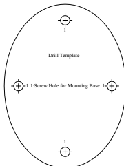
Рисунок 2-5 Шаблон крепления
