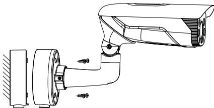
Рисунок 2-7 Установка камеры
