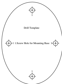
Рисунок 2-1 Шаблон крепления
