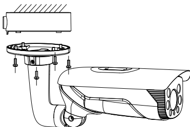
Рисунок 2-3 Установка камеры
