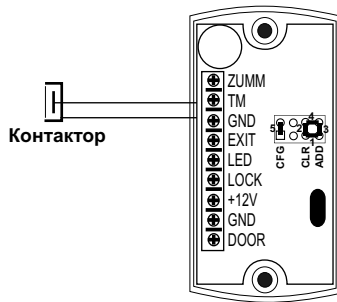
Рис.6 Подключение контактора
