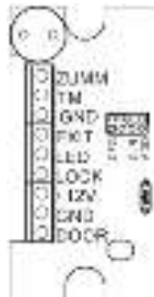
Рис.1 Габаритные размеры и расположение клемм
