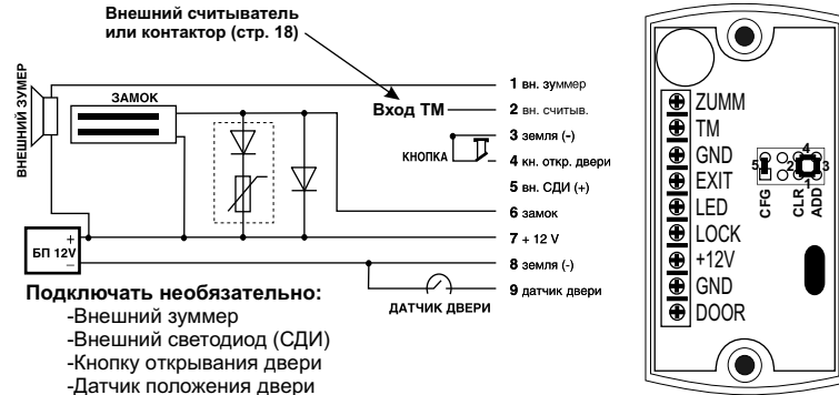
Рис. 3 Подключение внешних устройств
