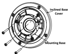
Рисунок 2-11 Установка монтажного основания
