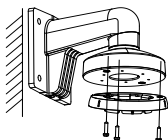
Рисунок 2-14 Установка монтажного основания на кронштейн для установки на стену
