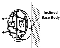
Рисунок 2-12 Фиксация корпуса наклонного основания на потолке/стене
