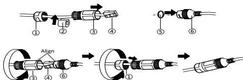
Рисунок 2-15 Установка гермоввода
