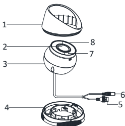
Рисунок 1-2 Внешний вид купольной камеры II типа
