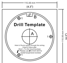
Рисунок 2-2 Шаблон крепления
