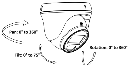
Рисунок 2-6 Регулировка угла наблюдения
