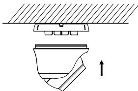
Рисунок 2-5 Установка корпуса камеры
