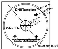
Рисунок 2-7 Шаблон крепления
