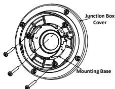
Рисунок 2-8 Установка монтажного основания
