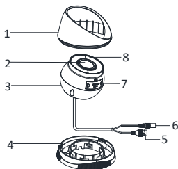
Рисунок 1-3 Внешний вид купольной камеры III типа
