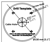
Рисунок 2-10 Шаблон крепления
