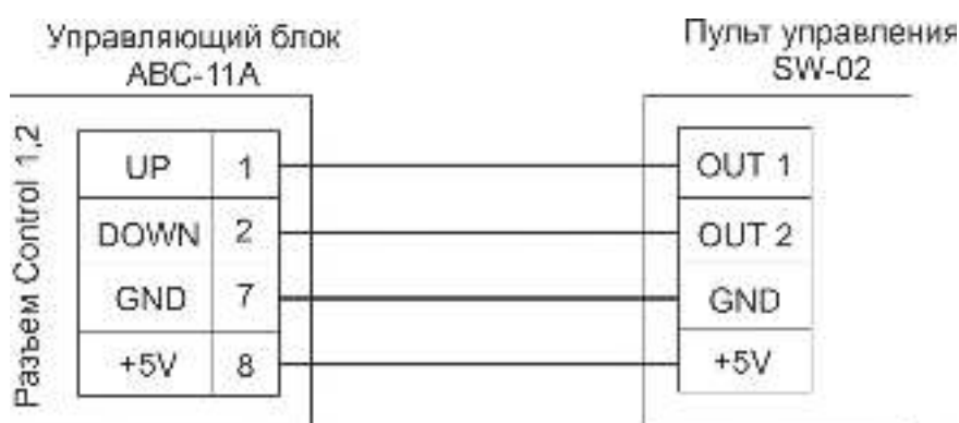
Рисунок 6.6.1.2 Схема подключения проводного ПДУ «SW-02»
