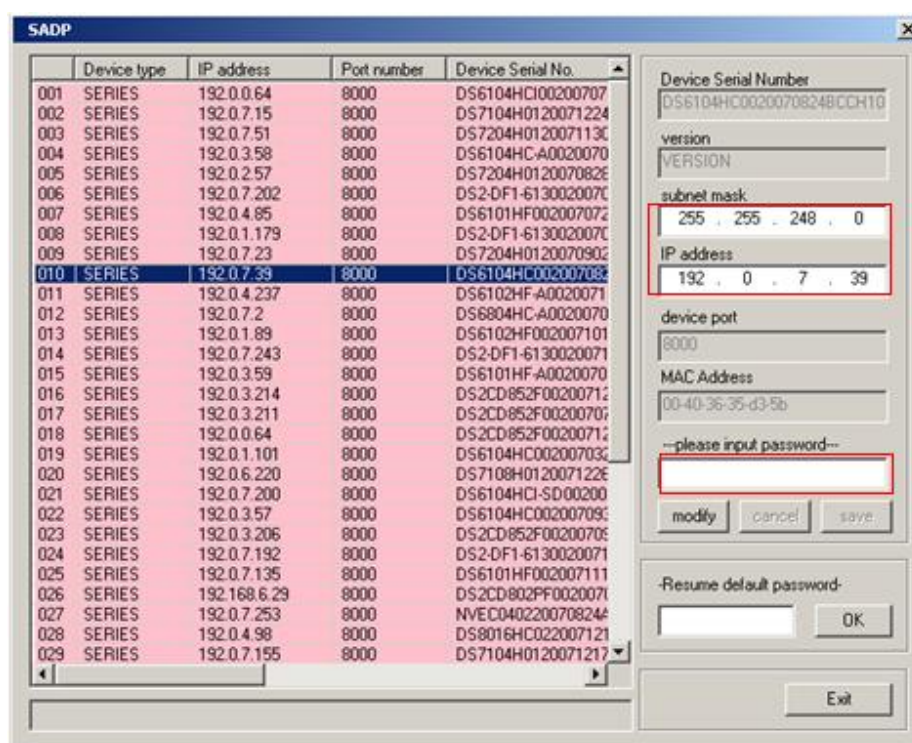
Рисунок 4.4.1 Поиск устройств в сети
