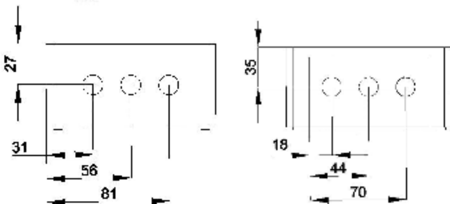
Для корпуса высотой 70мм
