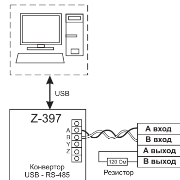
Рис.5 Схема подключения по RS-485.
