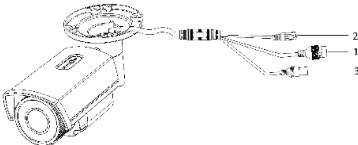
Рис. 2 Коммутационный кабель
