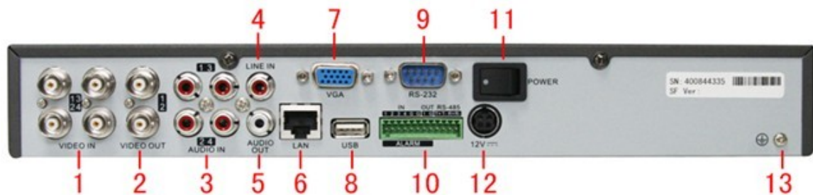
Рис 14. Задняя панель DS-7204HVI-ST
