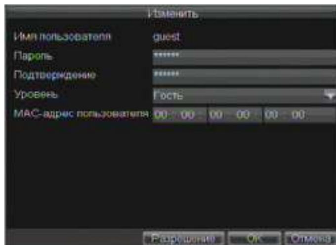
Рис. 9. Меню изменения учетной записи
