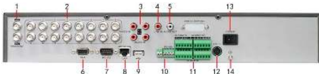
Figure 17. Задняя панель DS-7216HVI-ST
