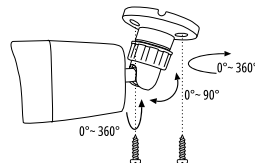
Рис. 3 Установка видеокамеры STAR ×3
