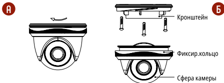
Рис. 1 Установка видеокамеры STAR ×2
