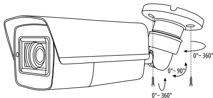
Рис. 5 Установка и регулировка обзора видеокамеры STAR ×8
