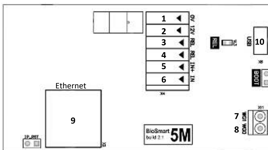
Рисунок 2 – плата контроллера
