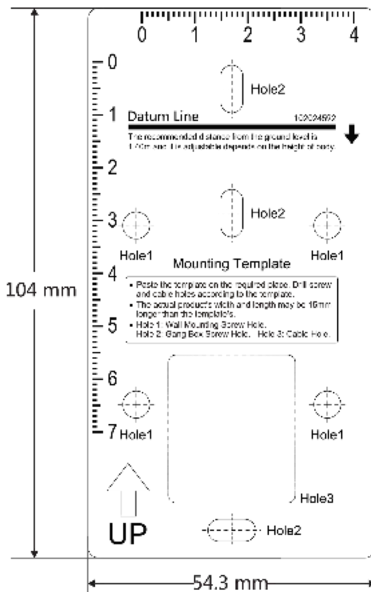
Рисунок 3-7. Монтажный шаблон
