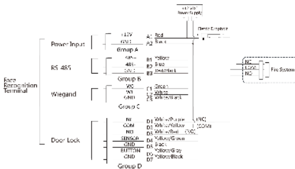
Рисунок 4-5. Подключение устройства
