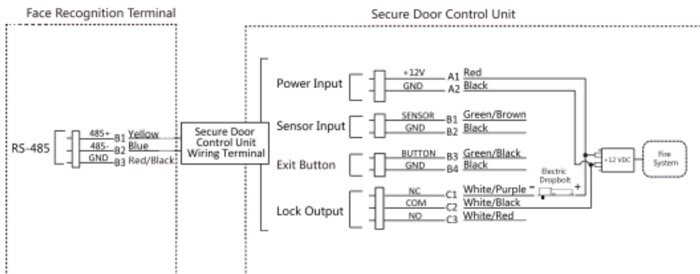
Рисунок 4-4. Подключение к модулю безопасности двери
