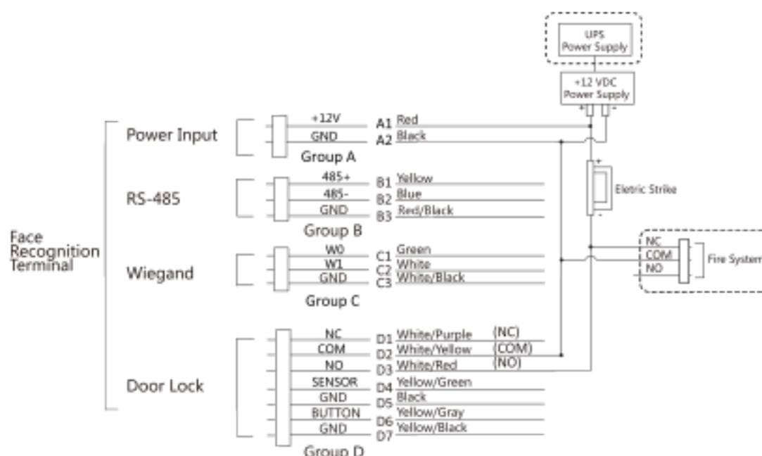
Рисунок 4-7. Подключение устройства
