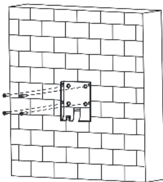
Рисунок 3-8. Установка монтажной платы
