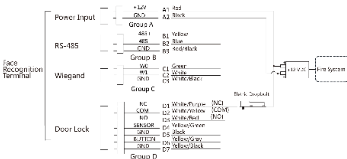
Рисунок 4-3. Подключение устройства
