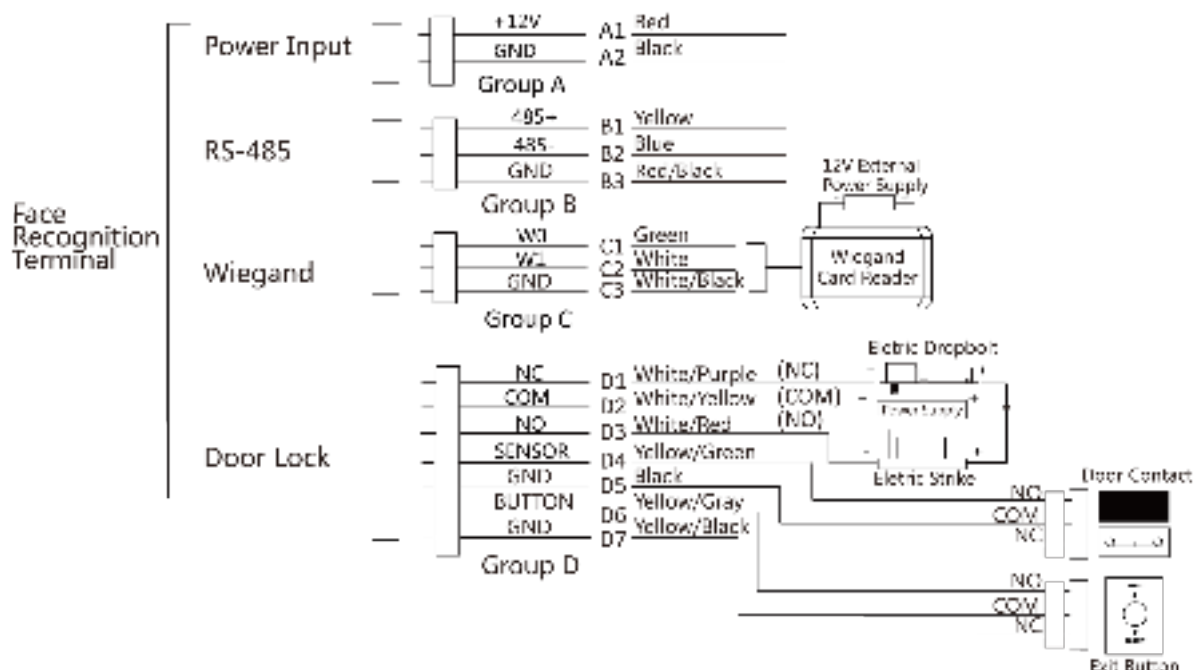
Рисунок 4-1. Подключение устройства
