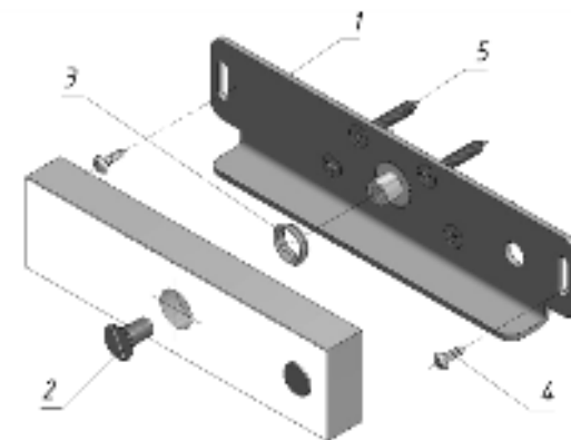
Рисунок 2 – Якорь с комплектом крепления 180Р
