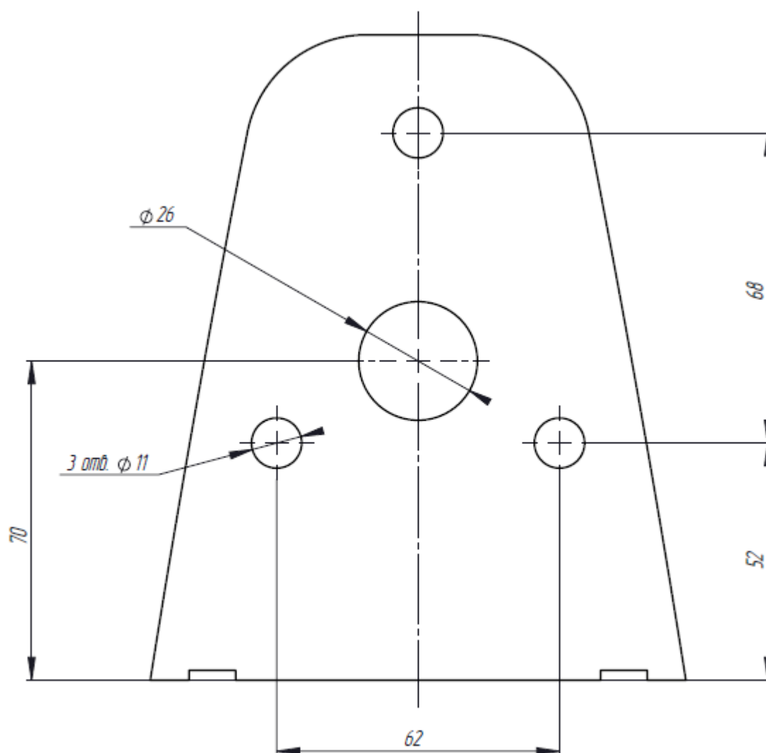
Рисунок 2 – Установочные размеры площадки
