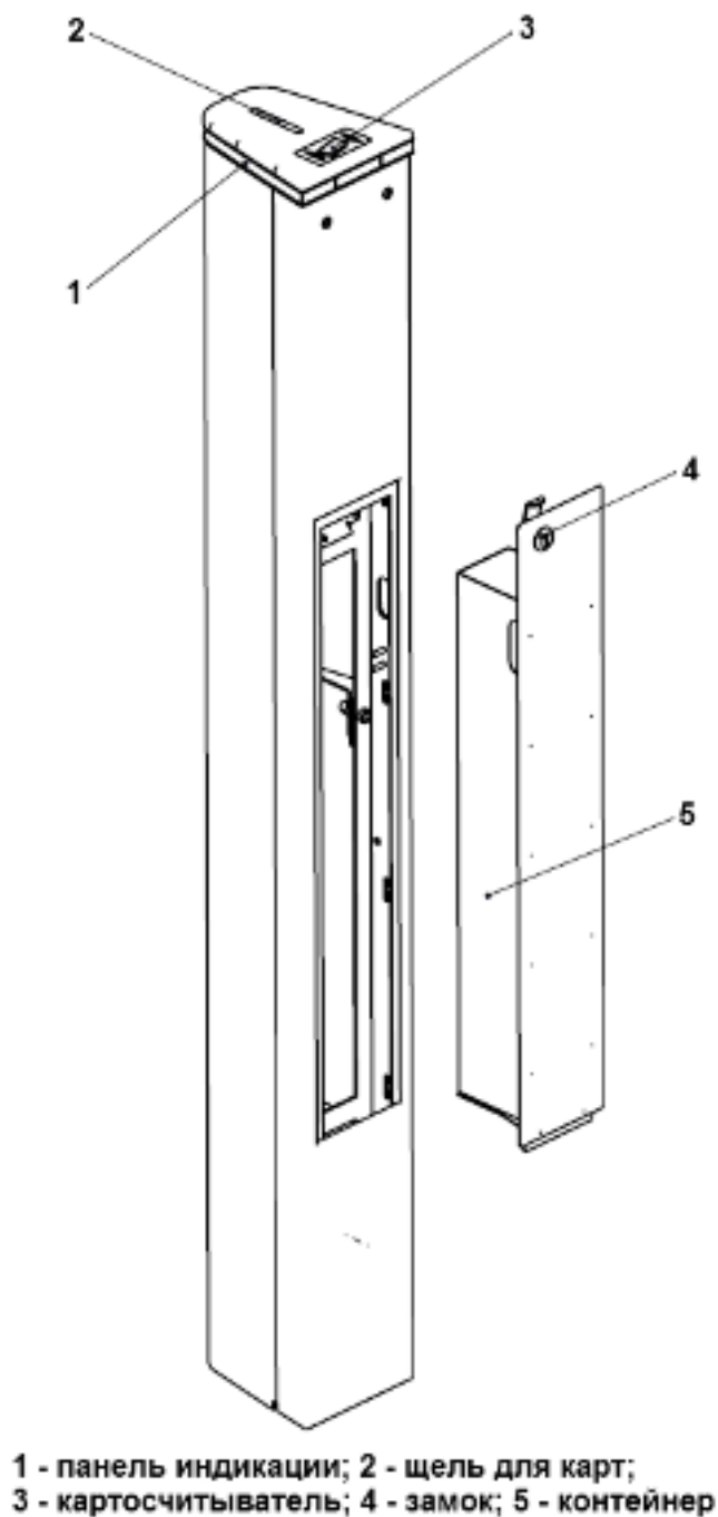
Рисунок 3 – Общий вид стойки картоприемника
