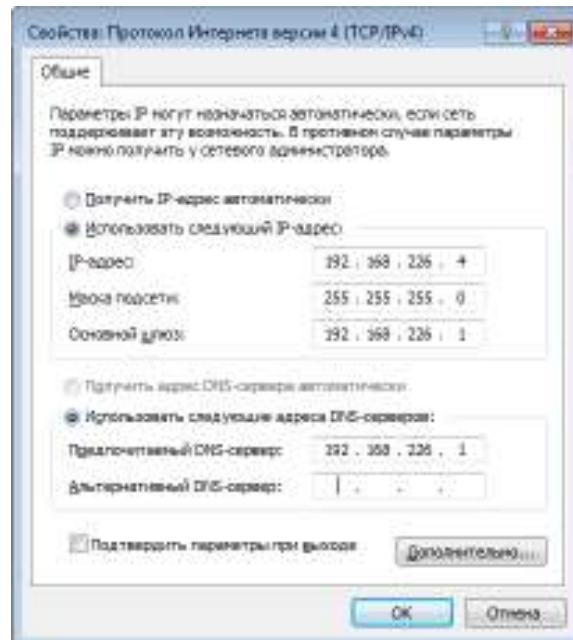
Рис. 6.4. Настройки IP-протокола
